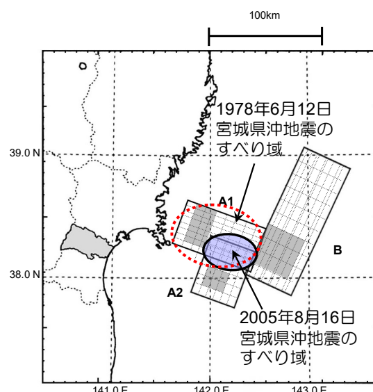
図 1 想定宮城県沖地震のすべり域
